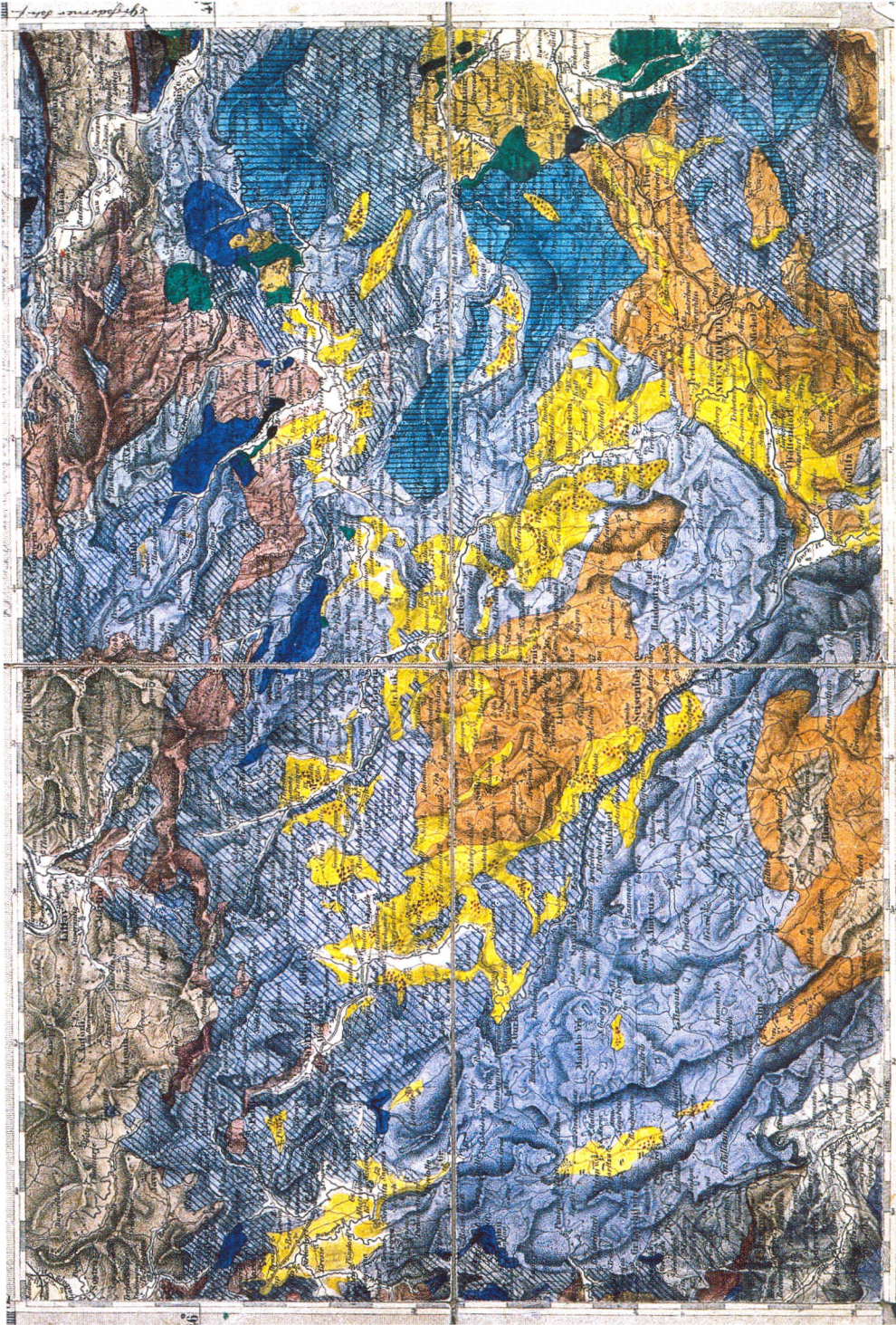
Sl. 6. Rokopisna geološka karta okolice Novega mesta in Višnje Gore Abb. 6. Geologische Manuskriptkarte der Umgebungen von Neustadt und Weixelburg
